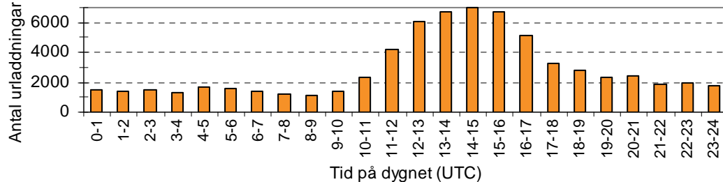
Figur 40. Dygnsvariation av antal urladdningar för Sverige samt landsdelar. Medelvärde för åren 2002-2009. Observera att tiden anges i UTC samt den avvikande skalan för Sverige-diagrammet. (svensk sommartid = UTC + 2 timmar, svensk normalt看 = UTC + 1 timme)
