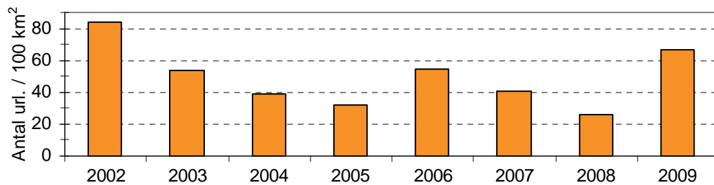
Figur 16. Antal urladdningar per areaenhet och år för hela landet samt för de fyra landsdelarna. Medelvärde baseras på samtliga beräkningsrutor (10 km x 10 km) inom respektive område.
